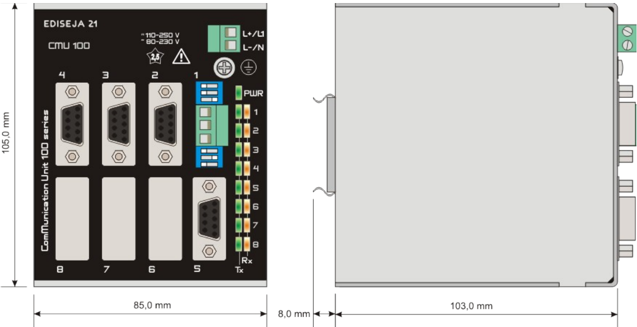
Picture 11: CMU 100 / 2.5.1.1.1.1-12 dimensions
