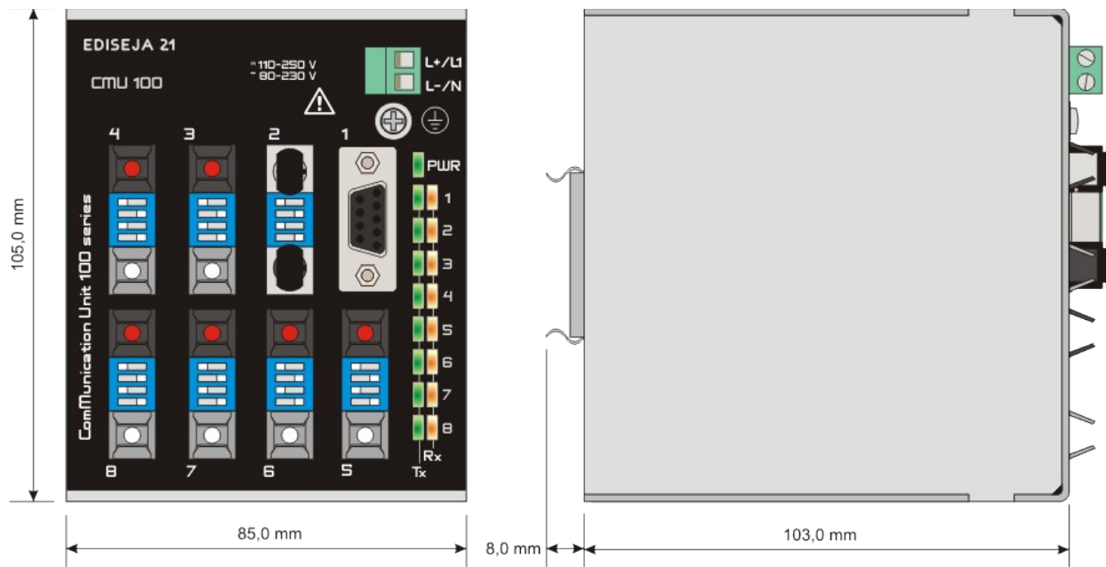
Picture 9: CMU 100 / x.1.6.P.P.P.P.P - 9 dimensions
