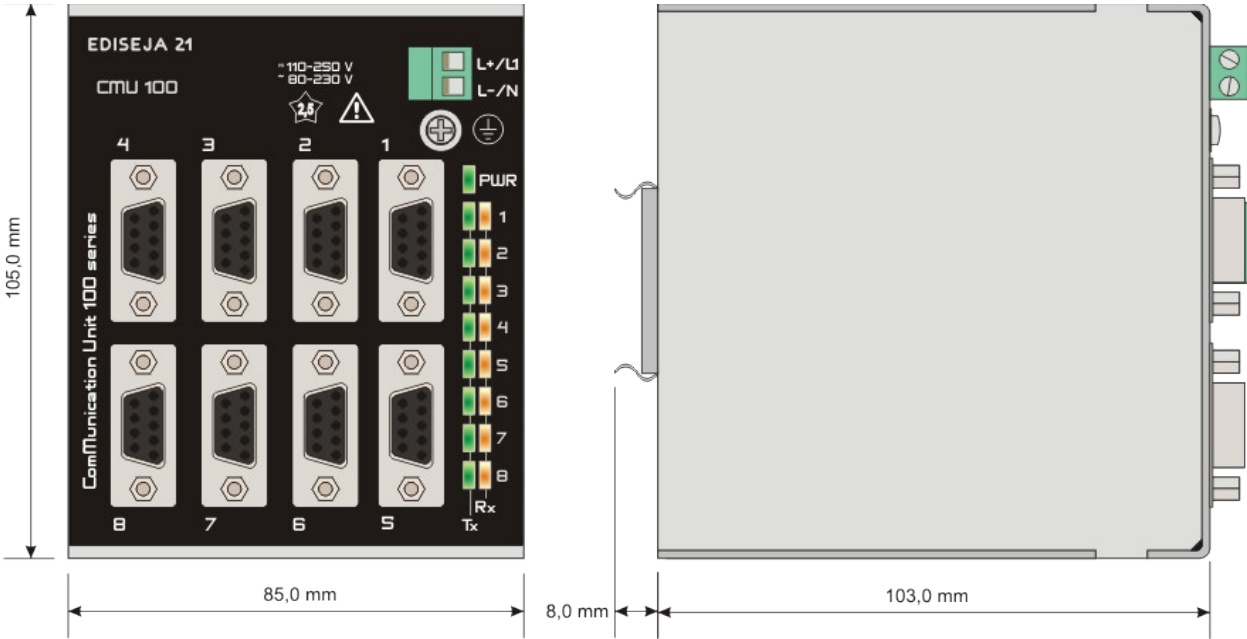
Picture 7: CMU 100 / 2.1.1.1.1.1.1 – 12 dimensions
