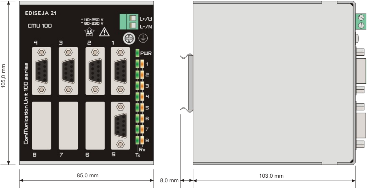
Picture 8: CMU 100 / 2.1.1.1.1.1-12 dimensions
